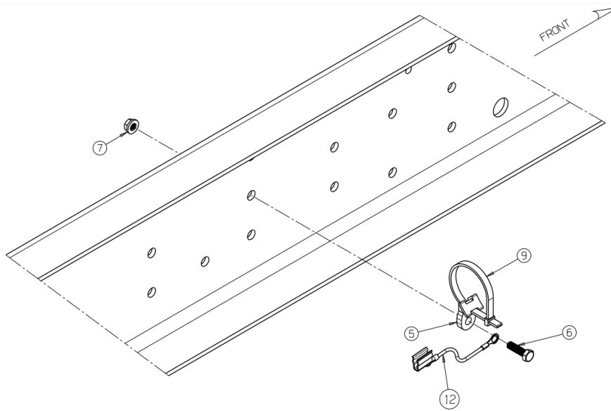
DETAIL E SCALE: 1:3
